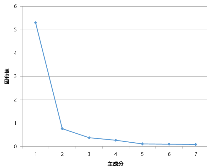
図2 主成分別の固有値
